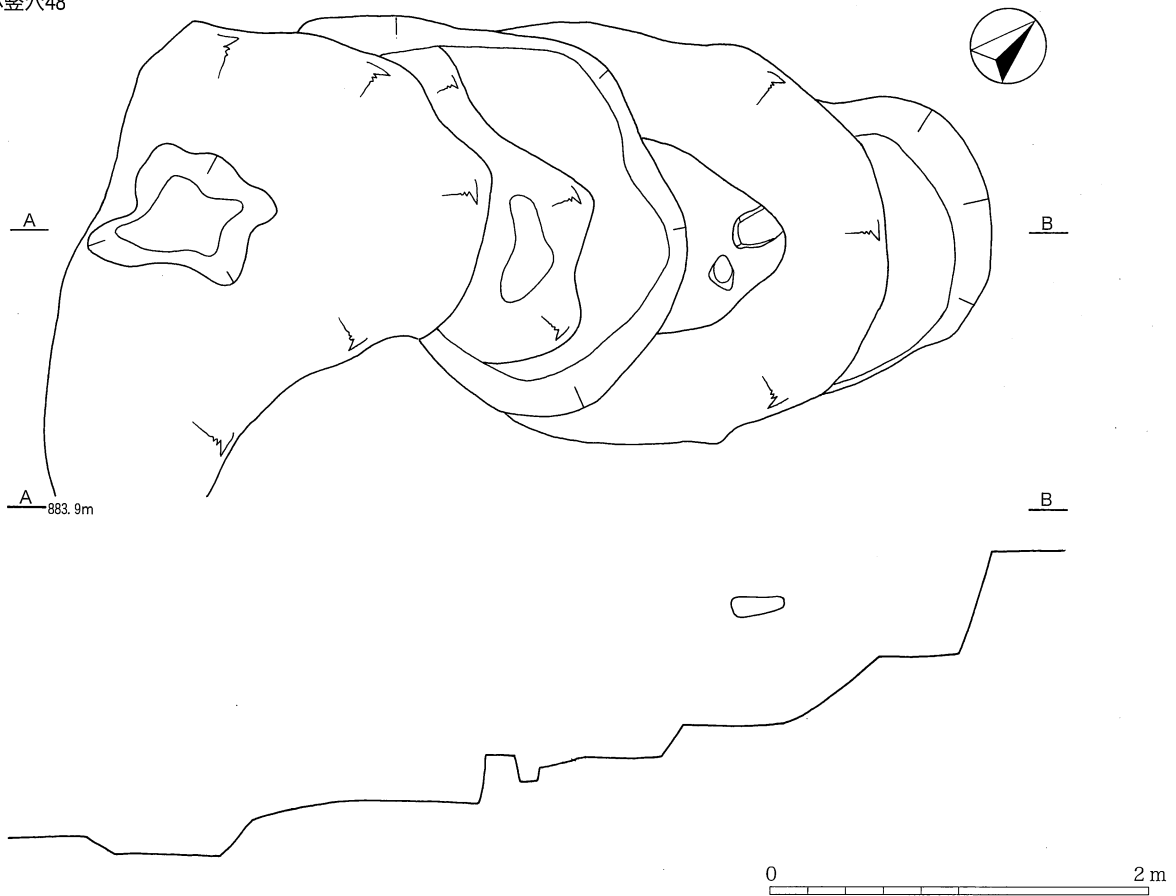
第142図 小豎穴47・48実測図 (1:40)
