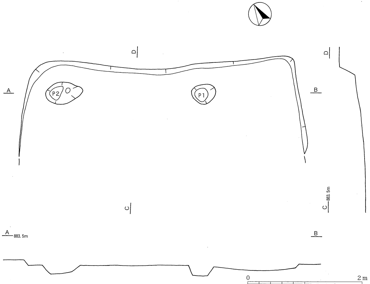
第141図 第20号竪穴住居址実測図（1：40）
