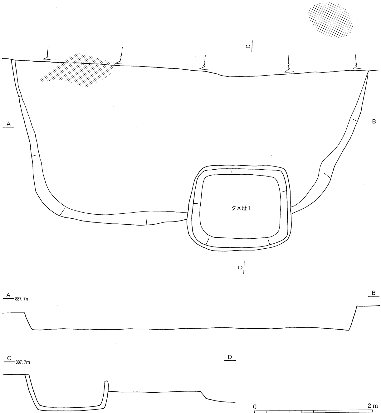
第140図 第4号竪穴住居址・タメ址実測図 (1:40)
