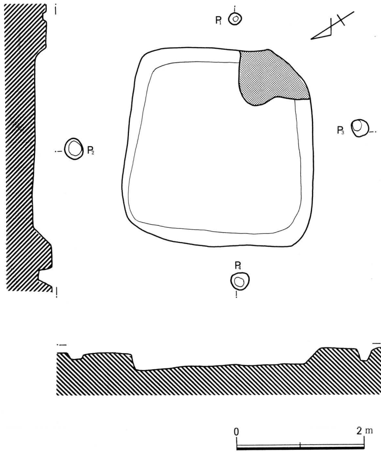
第5図 b号住居址 実測図 (1/60)
