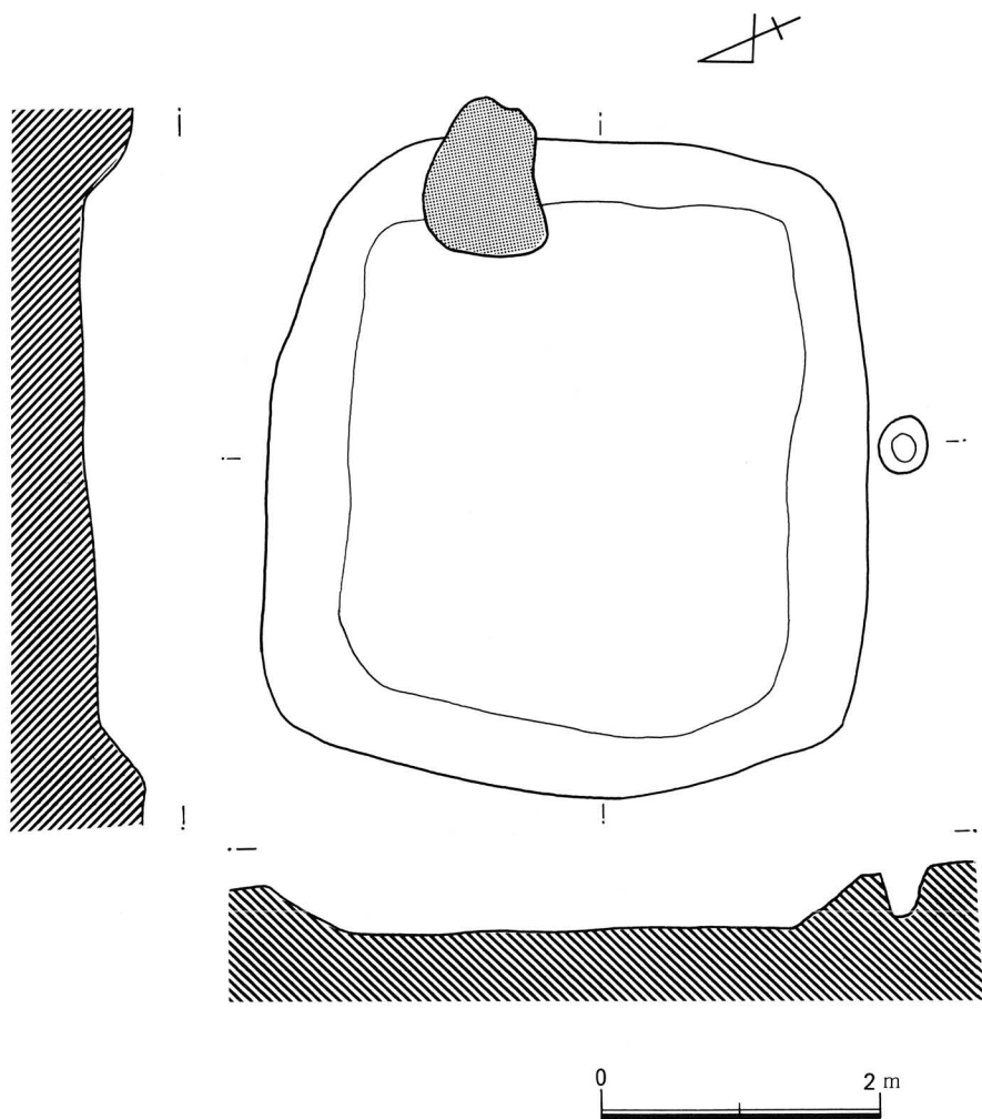
第6図 c号住居址 実測図 (1/60)
