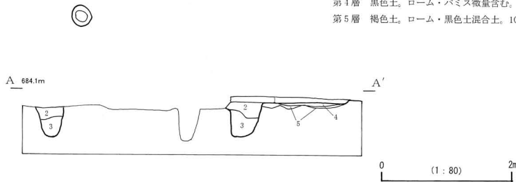
第8図 第4号住居址実測図
