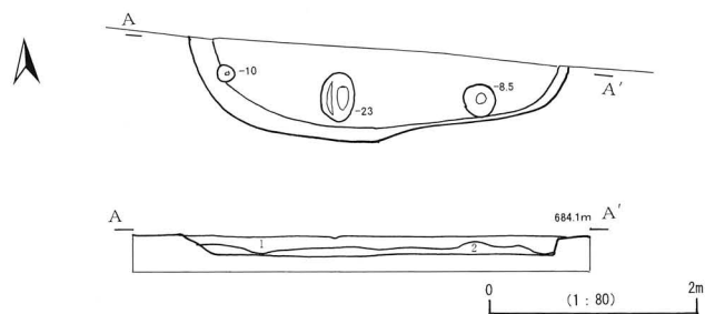
第13図 第12号住居址実測図
