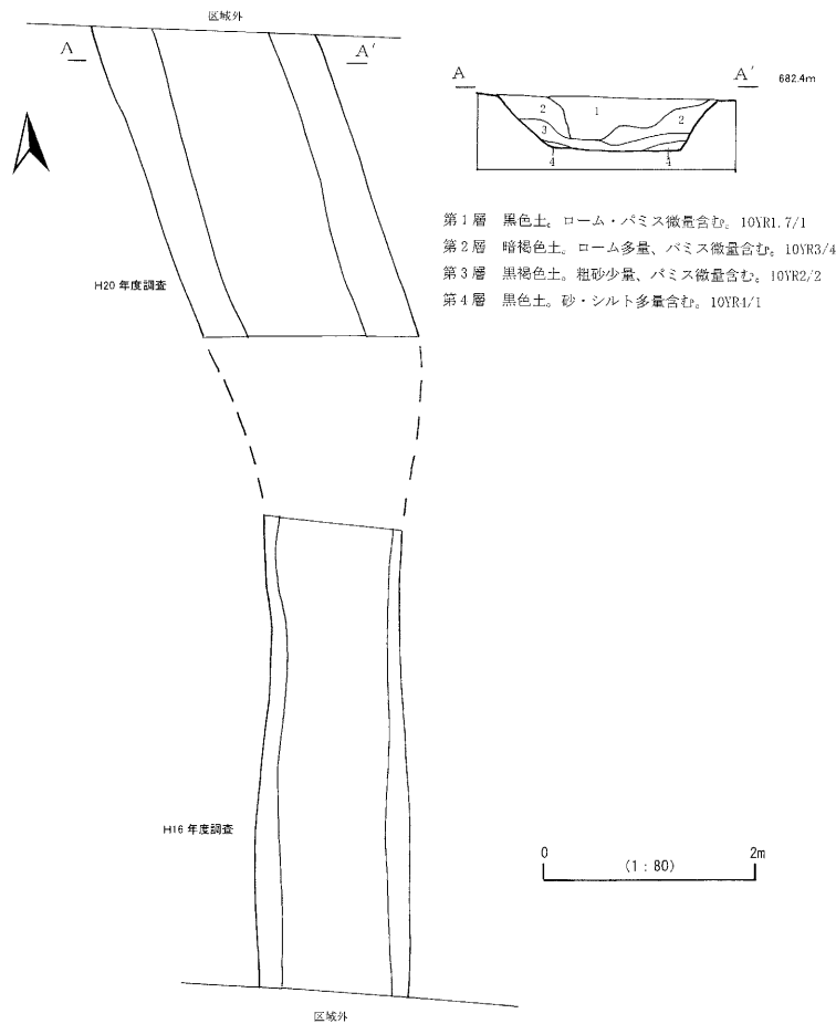
第15図 第4号溝址実測図
