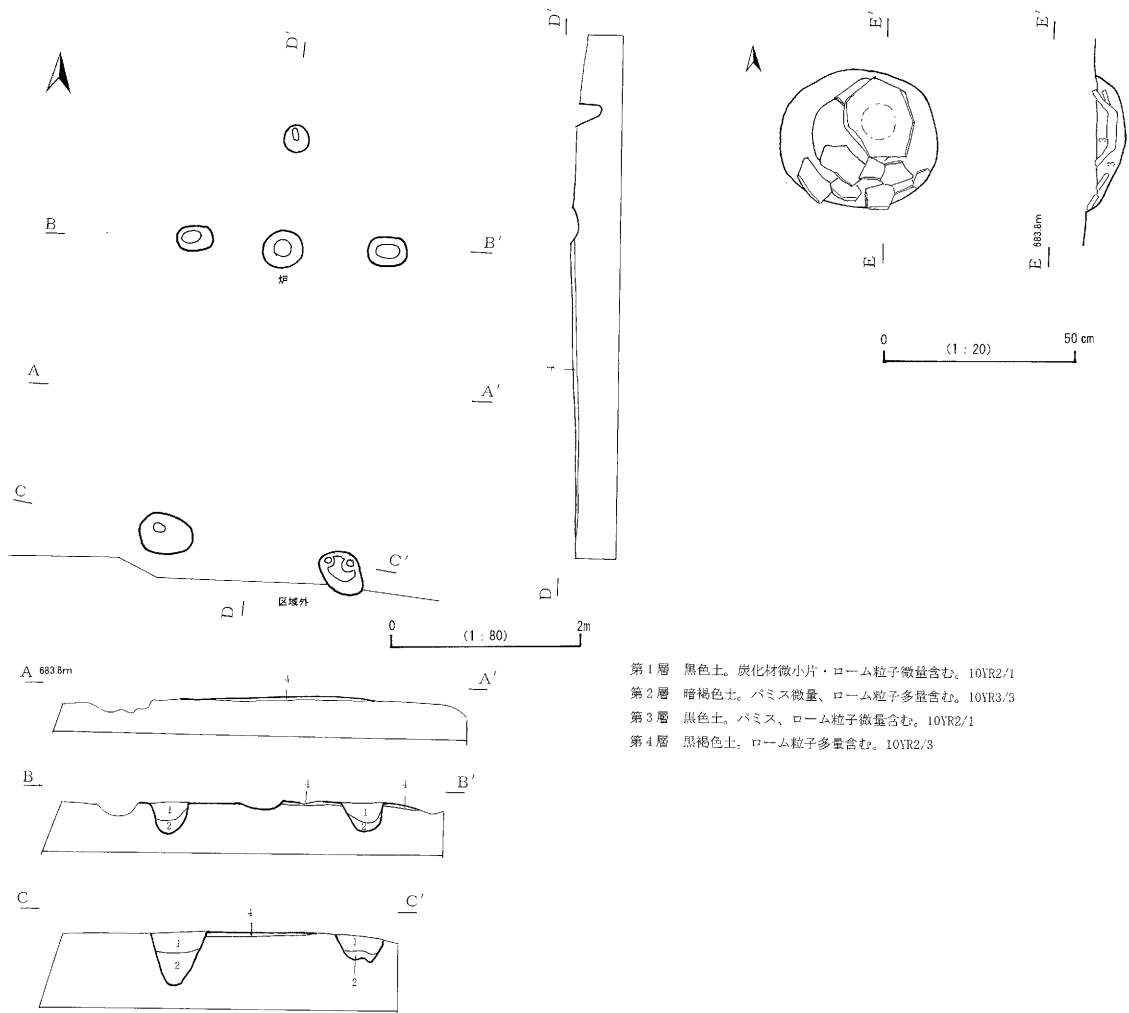
第5図 第1号住居址実測図
