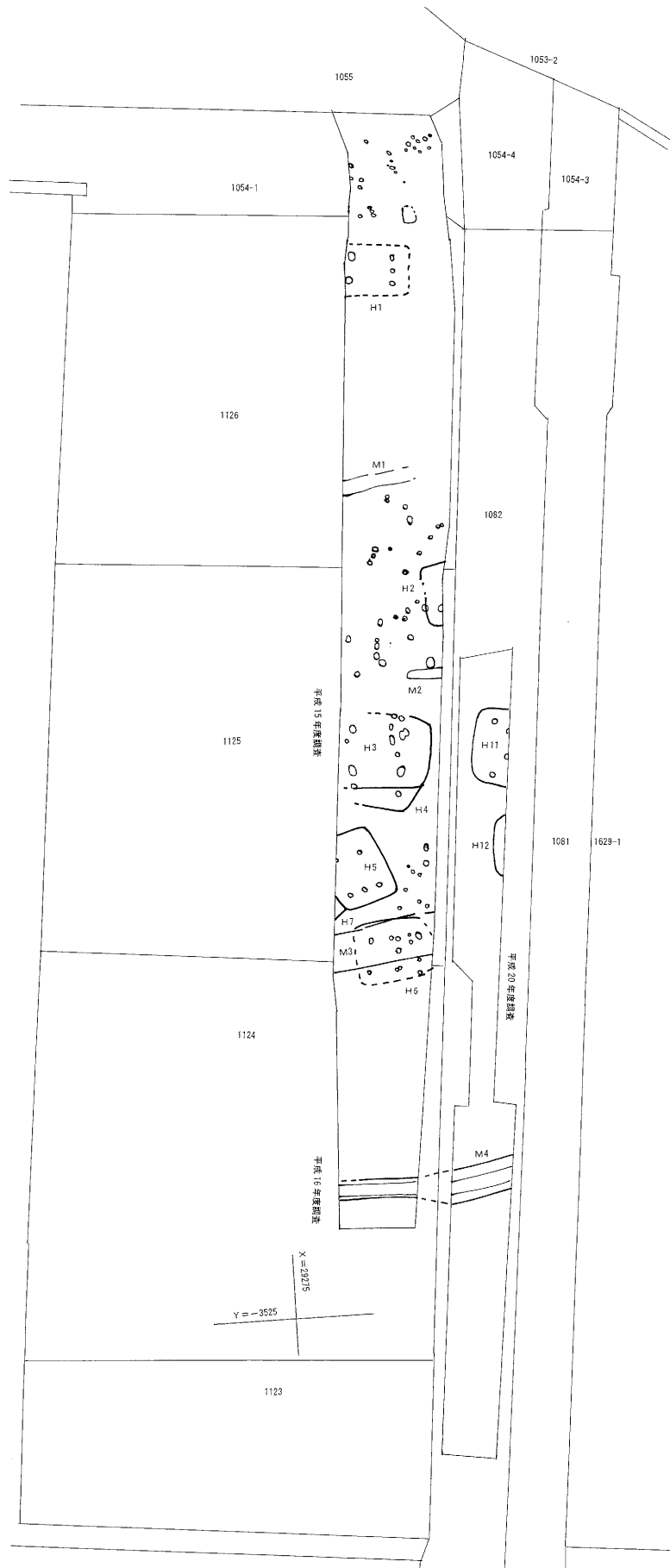
第4図 東側調査区全体図 (1:500)
