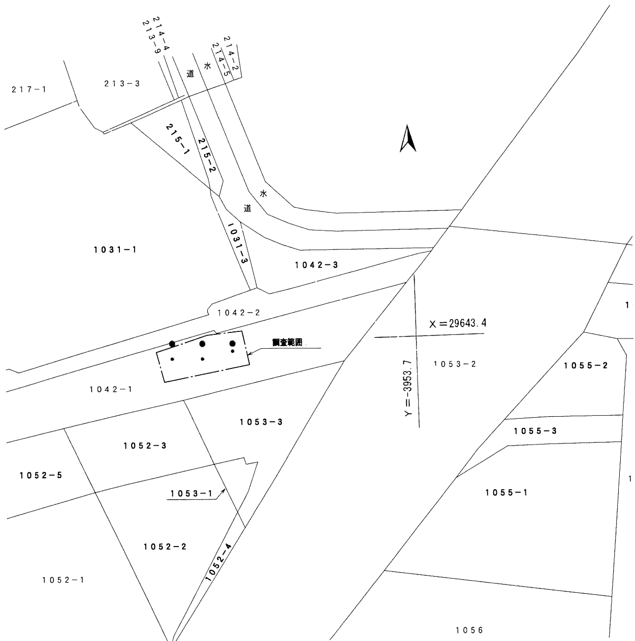
第16図 調査中央区全体図 (1 : 500)
