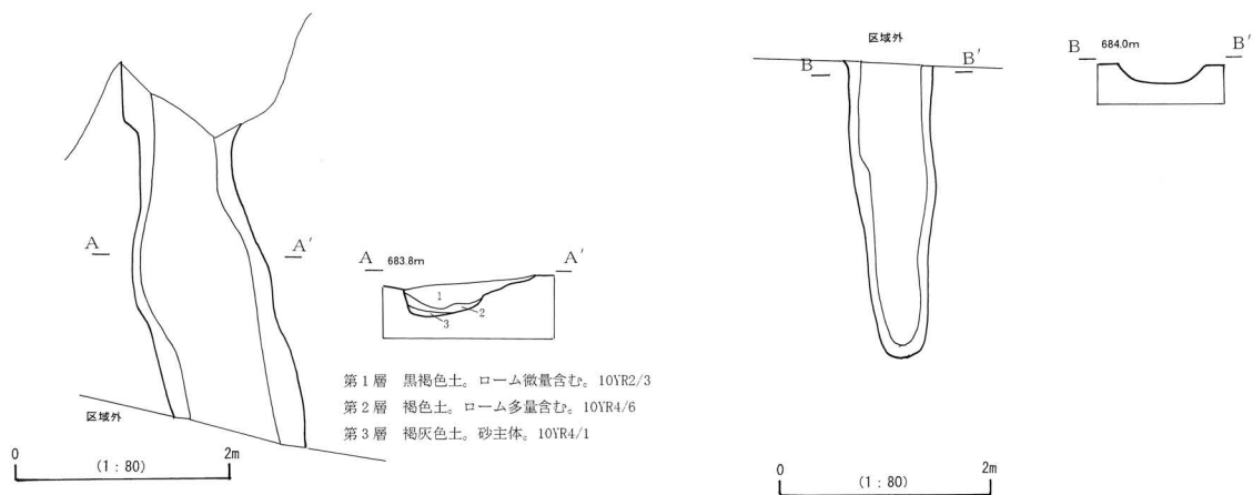
第14図 第1号・第2号溝址実測図 (左M1、右M2)
