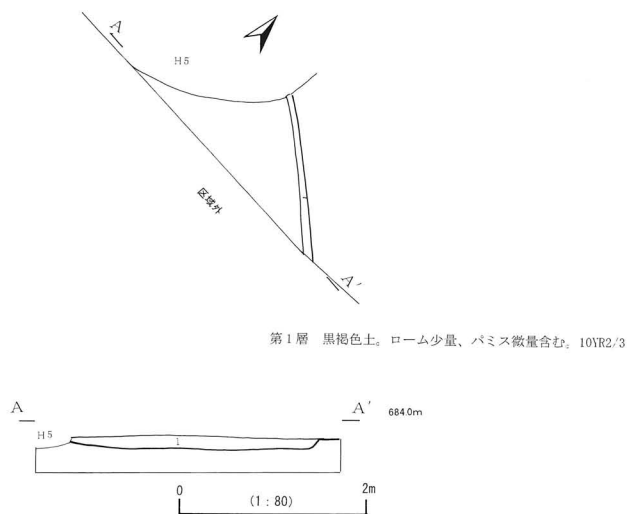
第11図 第7号住居址実測図
