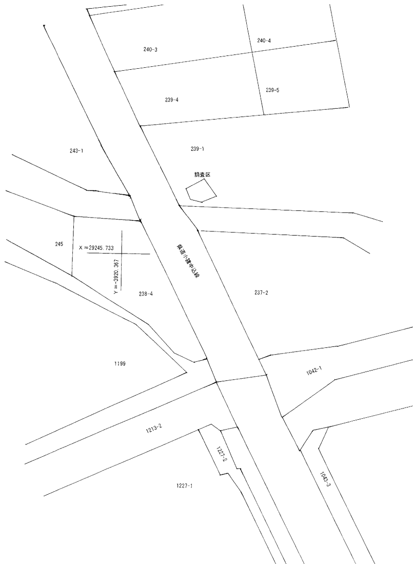
第18図 調査西区全体図 (1:500)
