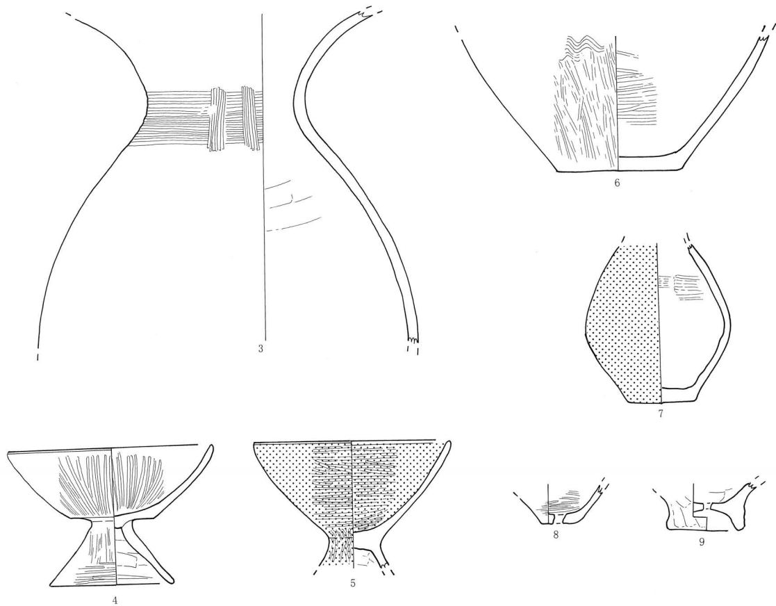
第21図 出土遺物実測図（2）網点は赤色塗彩範囲 1：4
