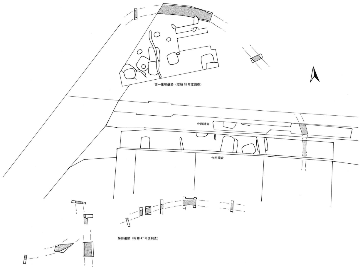
第3図 西一里塚遺跡調査全体図 (1:1,000)
