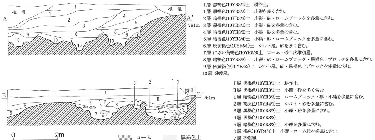
第3図 堀・溝址の土層堆積 (1:100)
