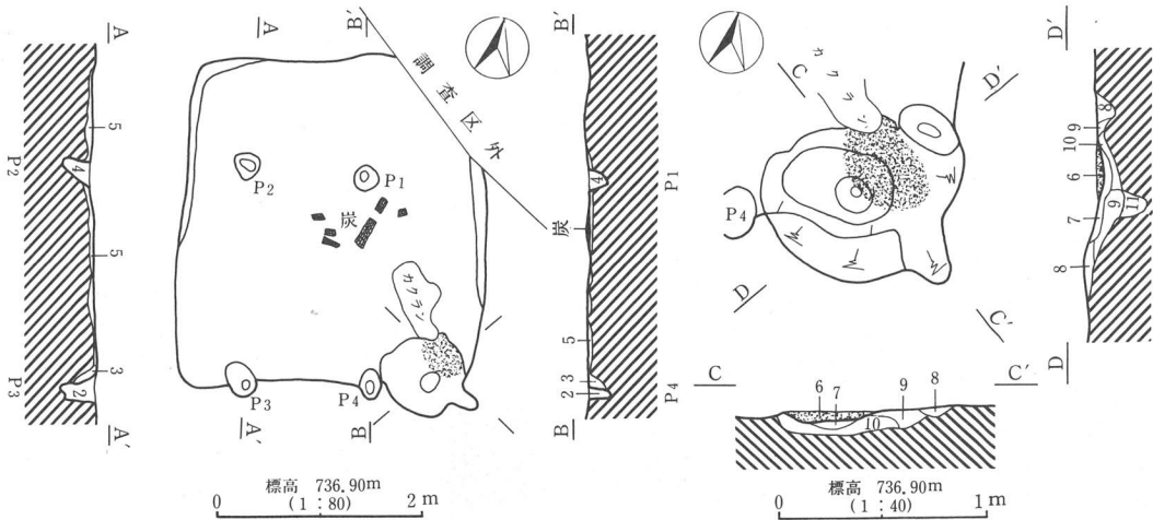
第166図 H45号住居址実測図
