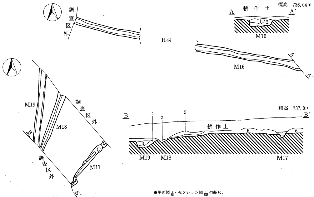
第167図 M16～M19号溝状遺構実測図
