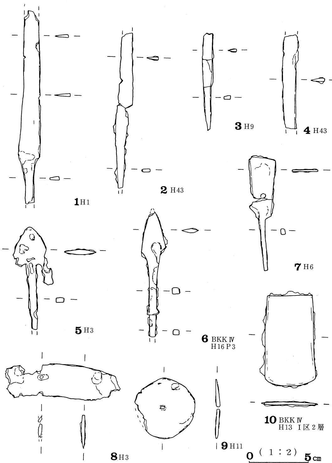
第182図 上久保田向遺跡出土鉄製品実測図(1)
