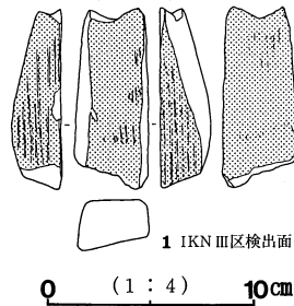
第180図 西首根遺跡出土石製品実測図
