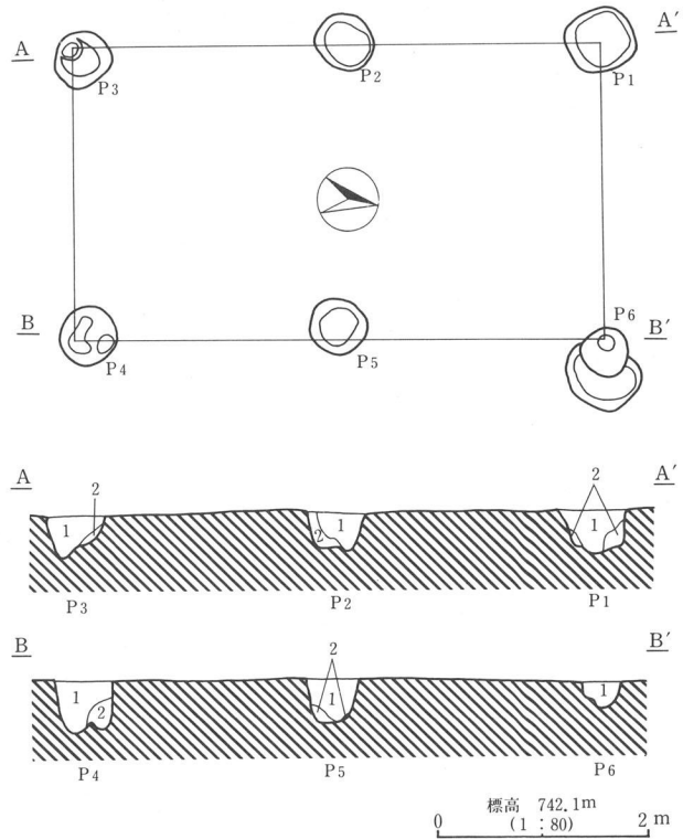
第171図 F18号掘立柱建物址実測図
