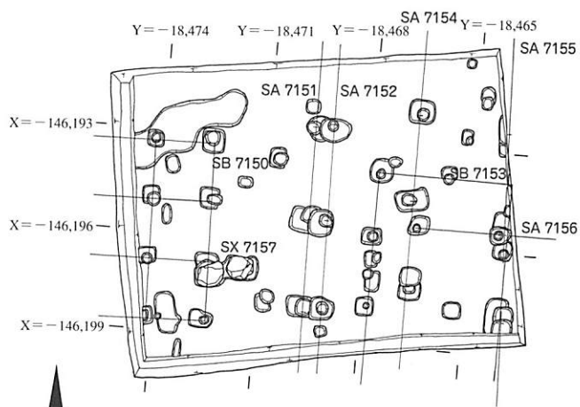
図95 第282-4次調査 遺構平面図 1:200
