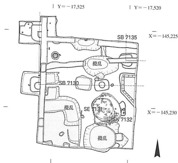
図94 第282-2次調査 遺構平面図 1:150
