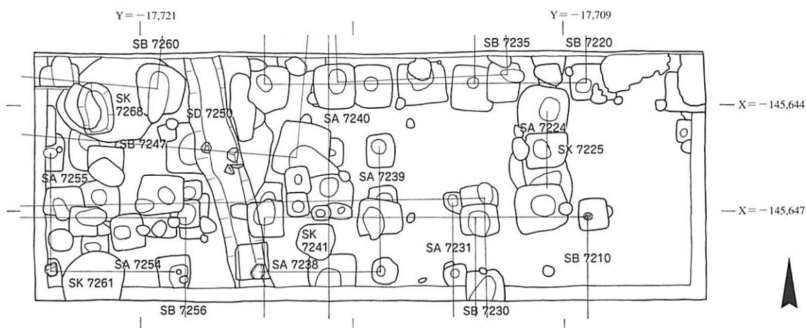
図76 第282-6次調査 遺構平面図 1:150
