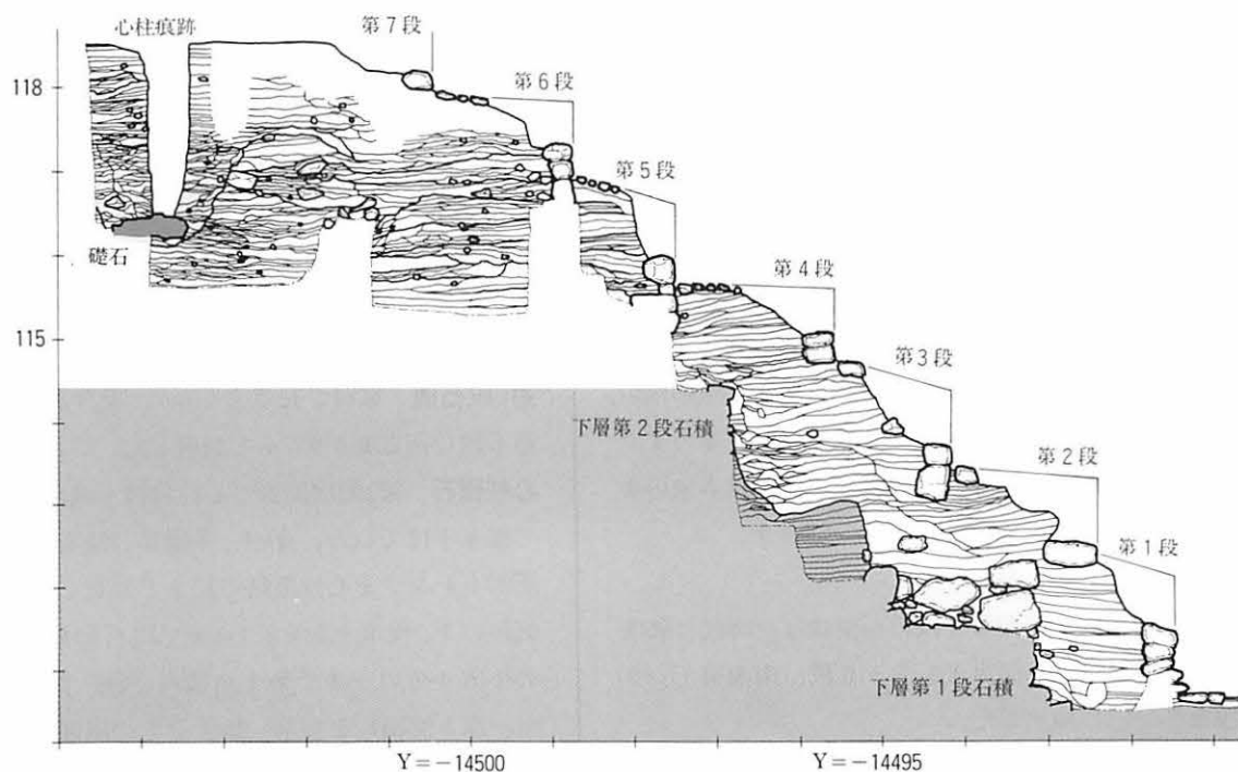
図44 頭塔断面模式図
