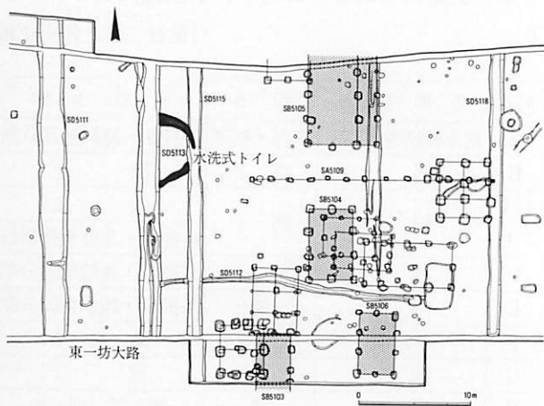
左京二条二坊の水洗式トイレ遺構図
