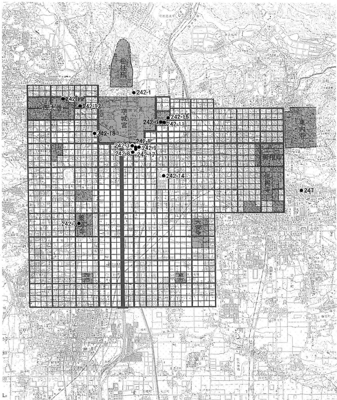
1993年度 平城京・京内寺院等の発掘調査位置図 1:50000
