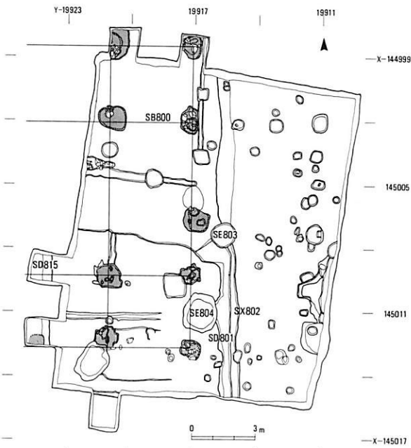
平城京第242-19次調査遺構図 1:250
