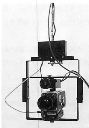
光軸を平行にしたときの カメラ架台
