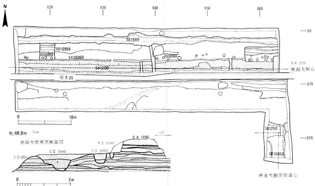
南面大垣調査遺構図
