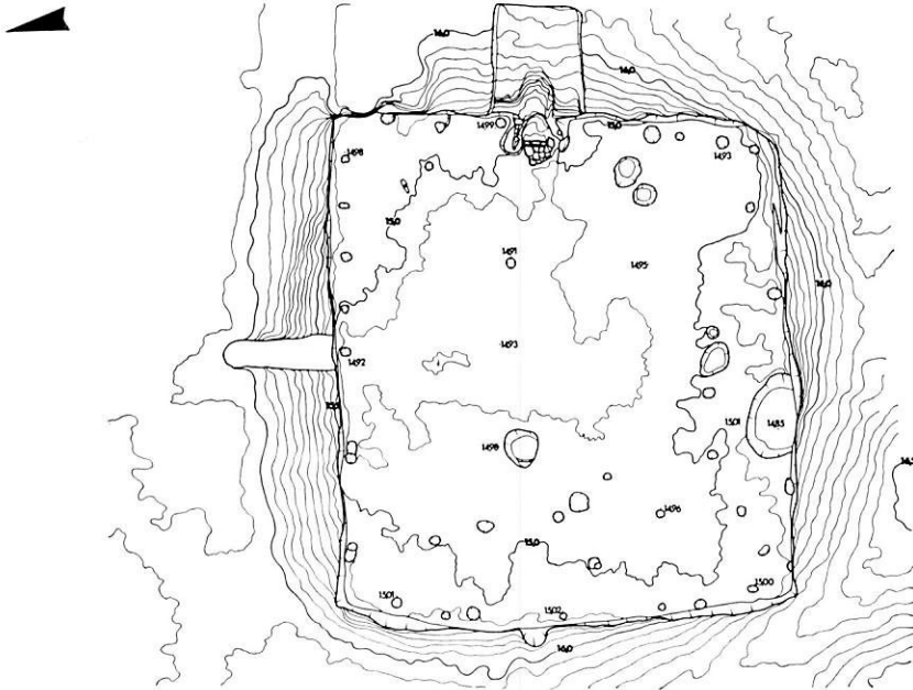
伊茶仁カリカリウス遺跡第1号堅穴写真測量図 縮尺1/100。等高線間隔5 cm。
