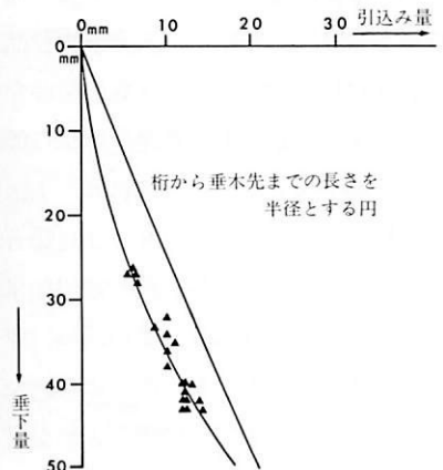
第3図 垂木先垂下量の経年変化
