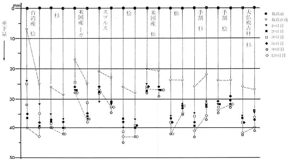
第4図 垂木先経年垂下量
