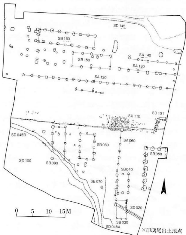
第7図 和陀摩寺遺構実測図
