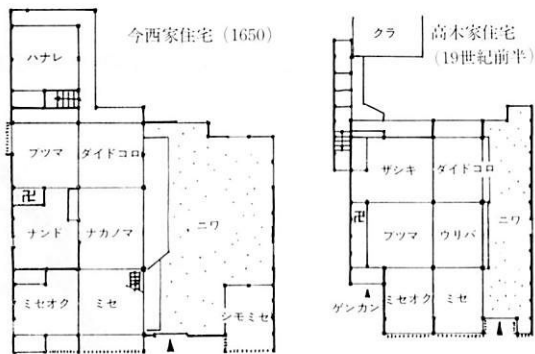
第1図 今井町民家平面図 6間取りの例
