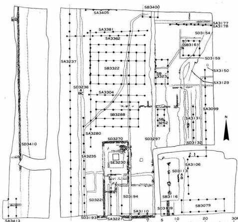
第7図 第22次調査南地区実測図
