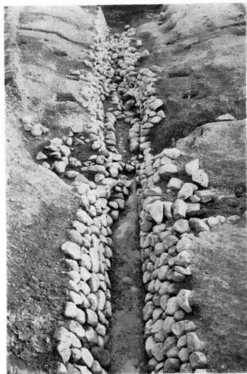
第4図 SD2700 玉石積大溝
