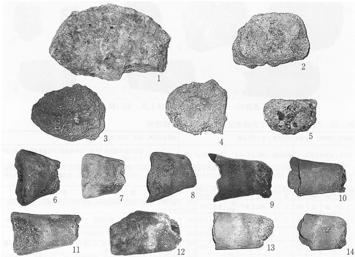
図-59 大県遺跡84-1次調査区出土鉄滓上面・羽口横 (S=約1/4)
