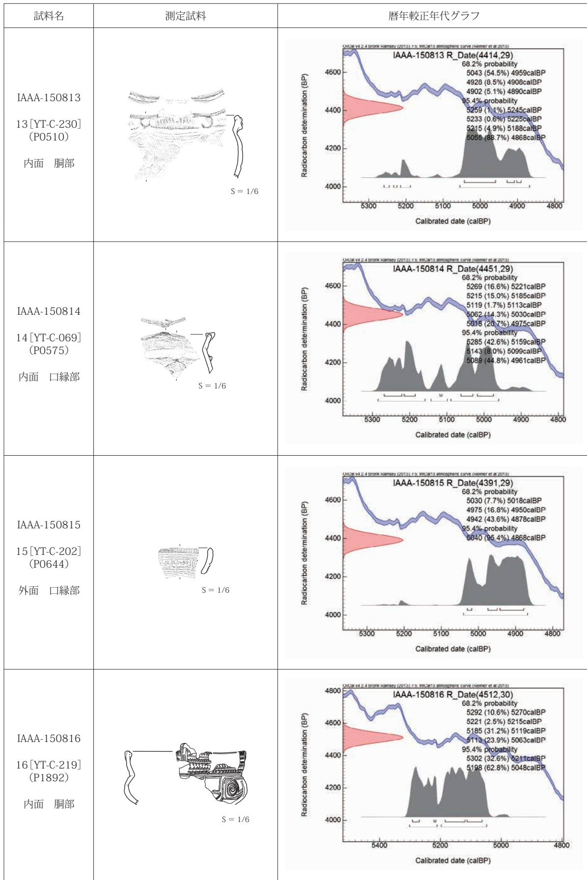
第 2-4 図 測定試料と暦年較正年代グラフ (4)
