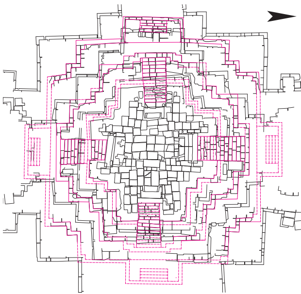
図79 ラテライト基壇平面図 1:200 (太線:残存部分、赤:残存部分から想定)
