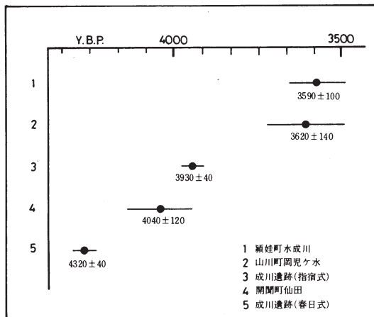
図－８ 開聞岳活動開始時期の ^{14}\text{C} 年代
