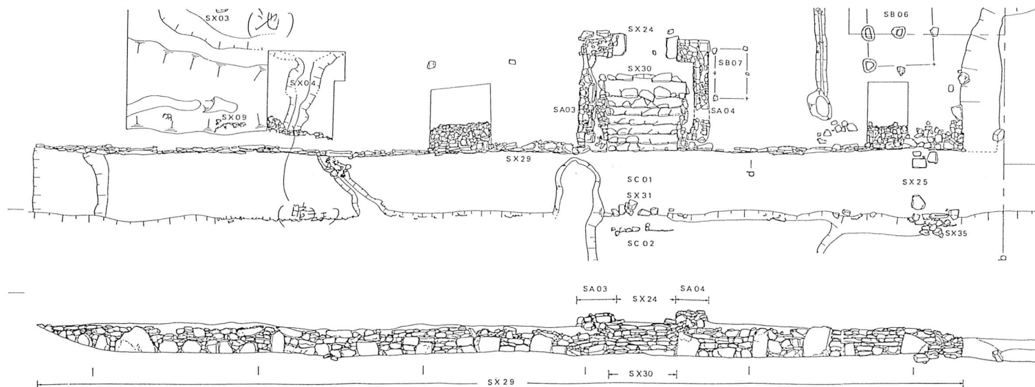
万徳院跡石垣実測平面図・立面図 (S≒1:250) (文献1)
