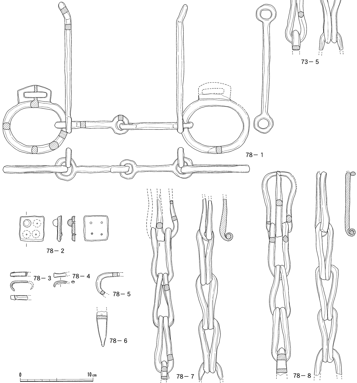
第 5 図 正知浦 2 号墳、小上野墓谷 2 号墳出土馬具 (S = 1 : 3)
