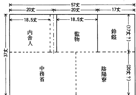
図7 中務省復原図
