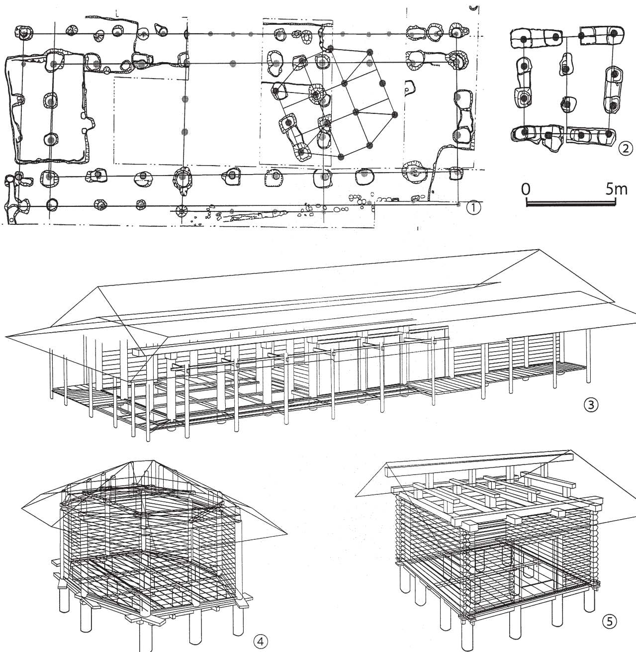
Fig.63 九間三面屋・八角倉・三間倉の復元
