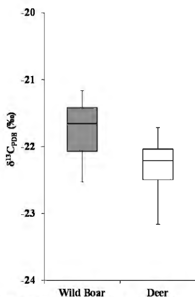
第 1 図 南貝塚出土動物遺存体の炭素同位体比
