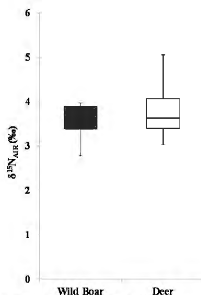
第 2 図 南貝塚出土動物遺存体の窒素同位体比
