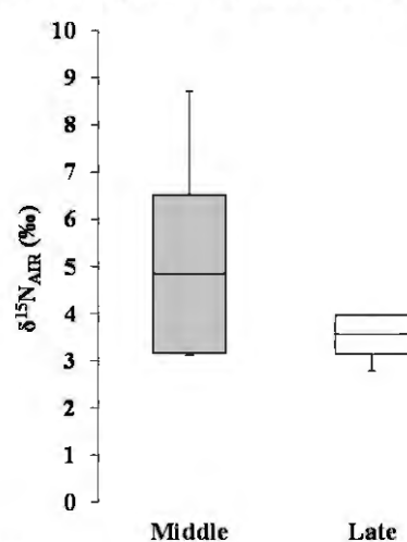
第 6 図 加曽利貝塚出土イノシシにおける 時代間の窒素同位体比
