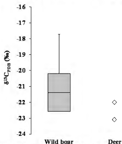
第 3 図 北貝塚出土動物遺存体の炭素同位体比
