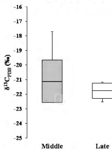
第 5 図 加曽利貝塚出土イノシシにおける 時代間の炭素同位体比
