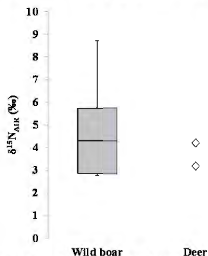
第 4 図 北貝塚出土動物遺存体の窒素同位体比
