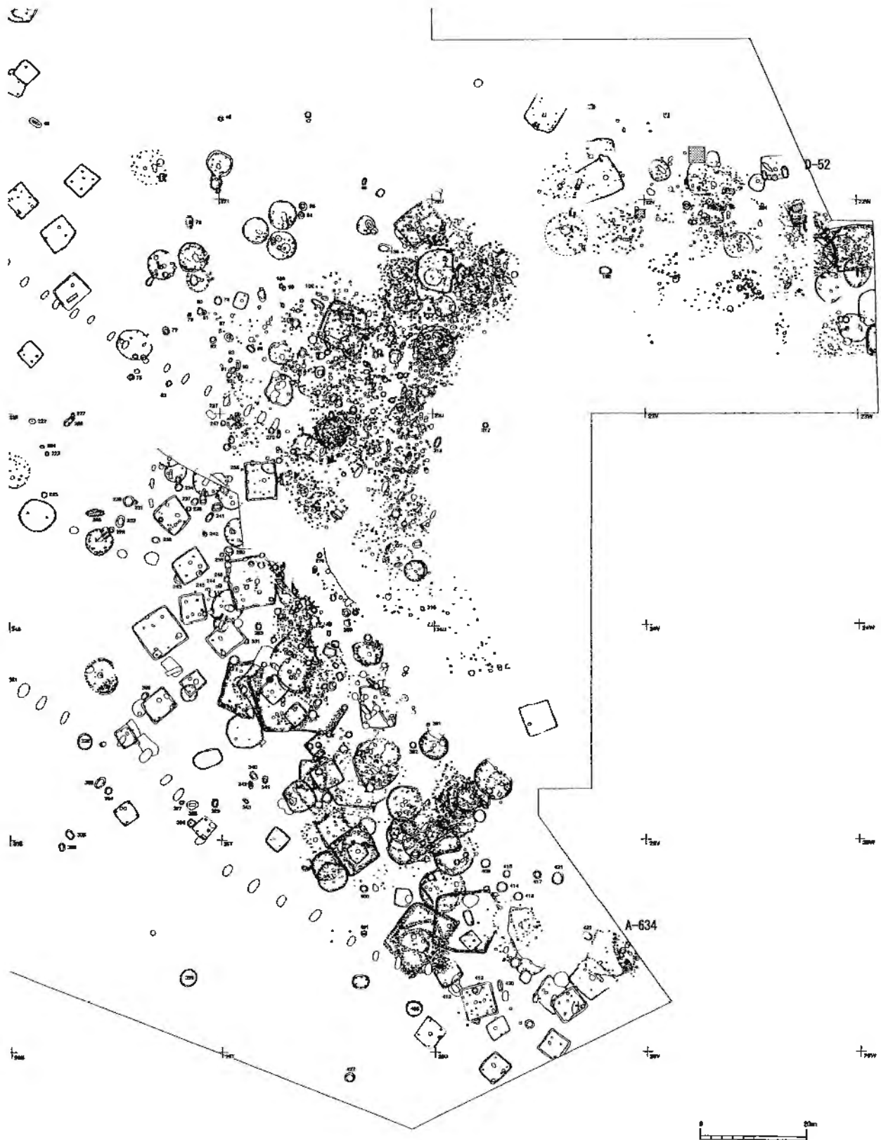
第 1 図 内野第 1 遺跡低地遺構配置図
