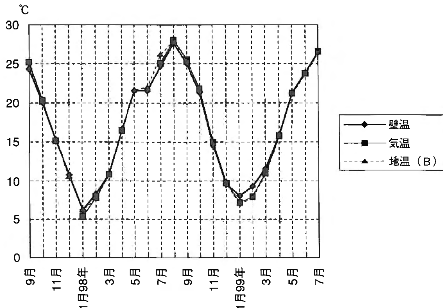
図5 気温、壁温、地温の季節変化の比較（1997年9月～1999年7月）
