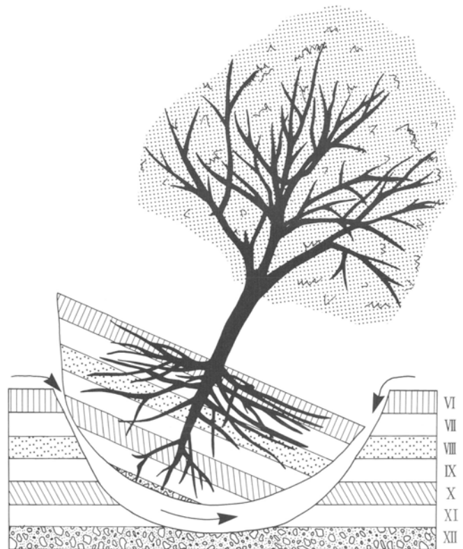
図4 根鉢の体積と表面積計算のための模式図(荻住1979より)
