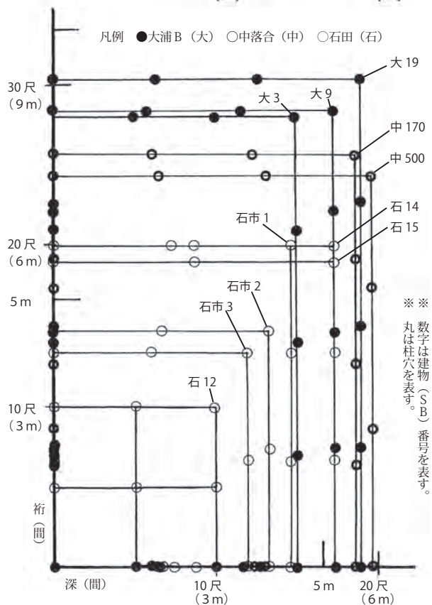
第8図 各遺跡のB類建物の平面形態図 (S = 1/100)
