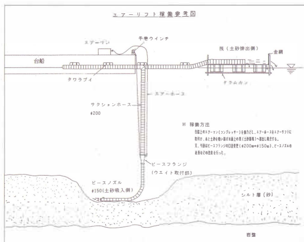
エアーリフト稼働参考図
