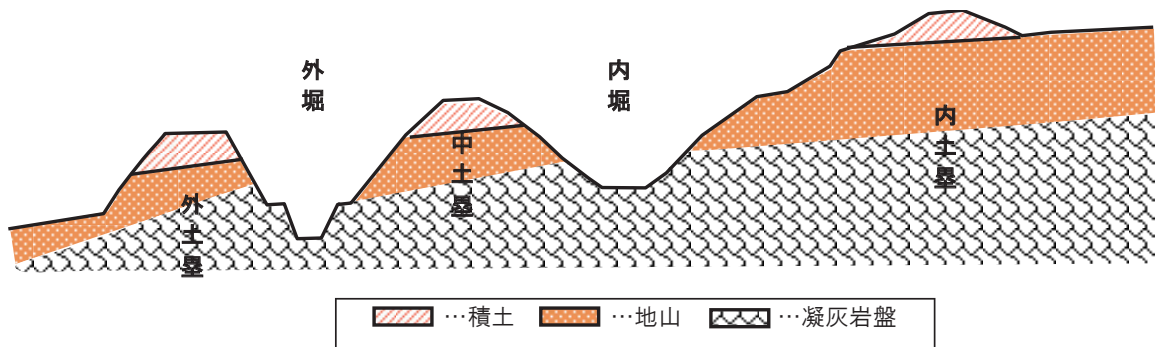
阿津賀志山防塁断面模式図(国道4号地区)
