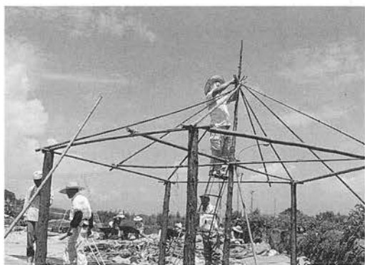
写真7 柱を組む
