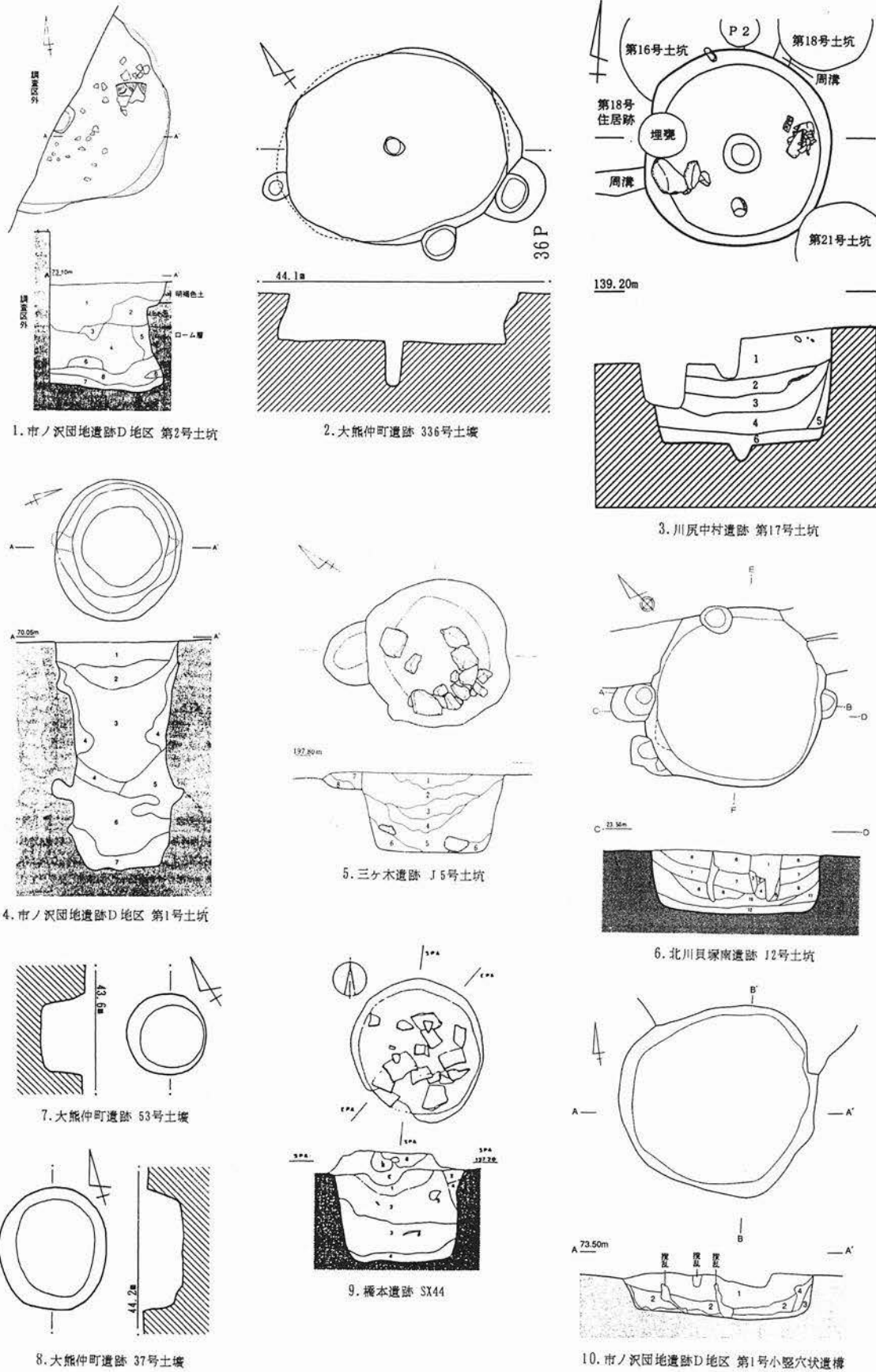
第8図 貯蔵穴〔S=1/60〕
