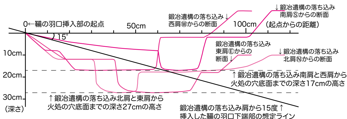
図 12 清郷遺跡鍛冶遺構の模式断面図 (1:10)
