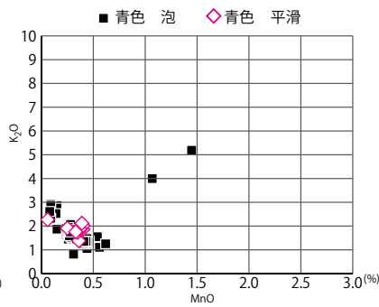
図3 K 2 O-MnO 図
