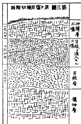
図1 佐藤傳蔵・若林勝邦(1894)の層序断面図
