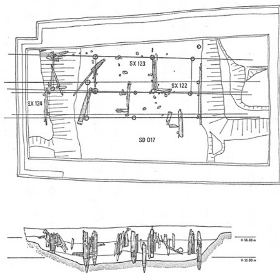
遺構平面・立面図
