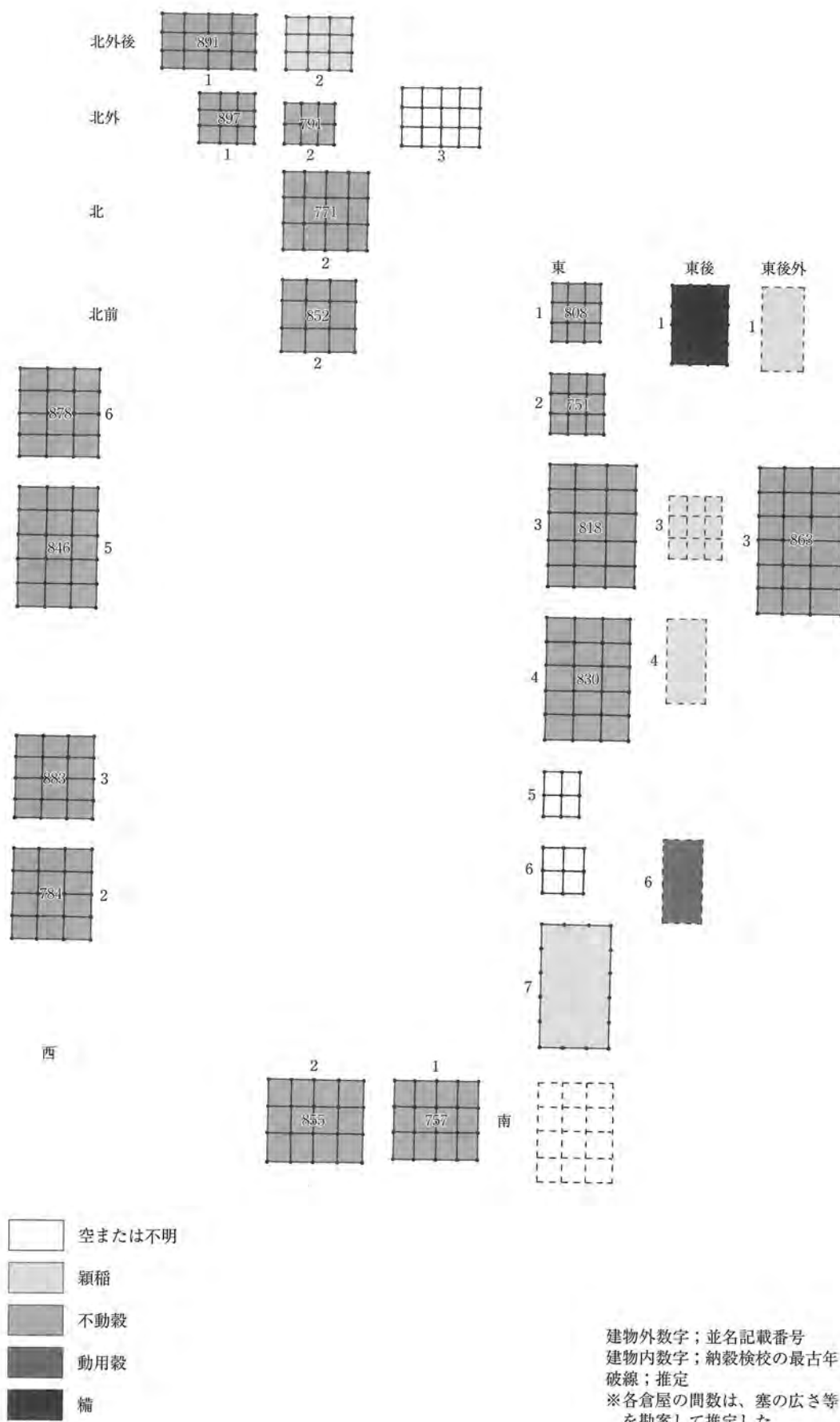
図5 「越中国官倉納穀交替記」による砺波郡意斐村の正倉規模と配置の復元
