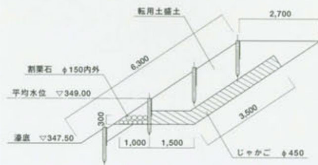
標準土留断面図
