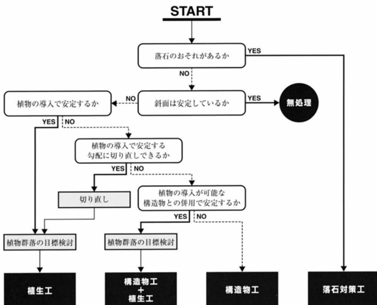
図-資2 斜面保護工選定の考え方及び手順
