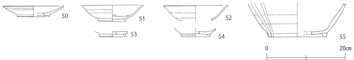
第2図 伊勢原市域出土灰釉葉陶器1 (S=1/6)
