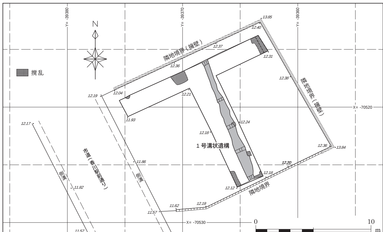
第 10 図 第 8 次調査遺構配置図 (1/200)
