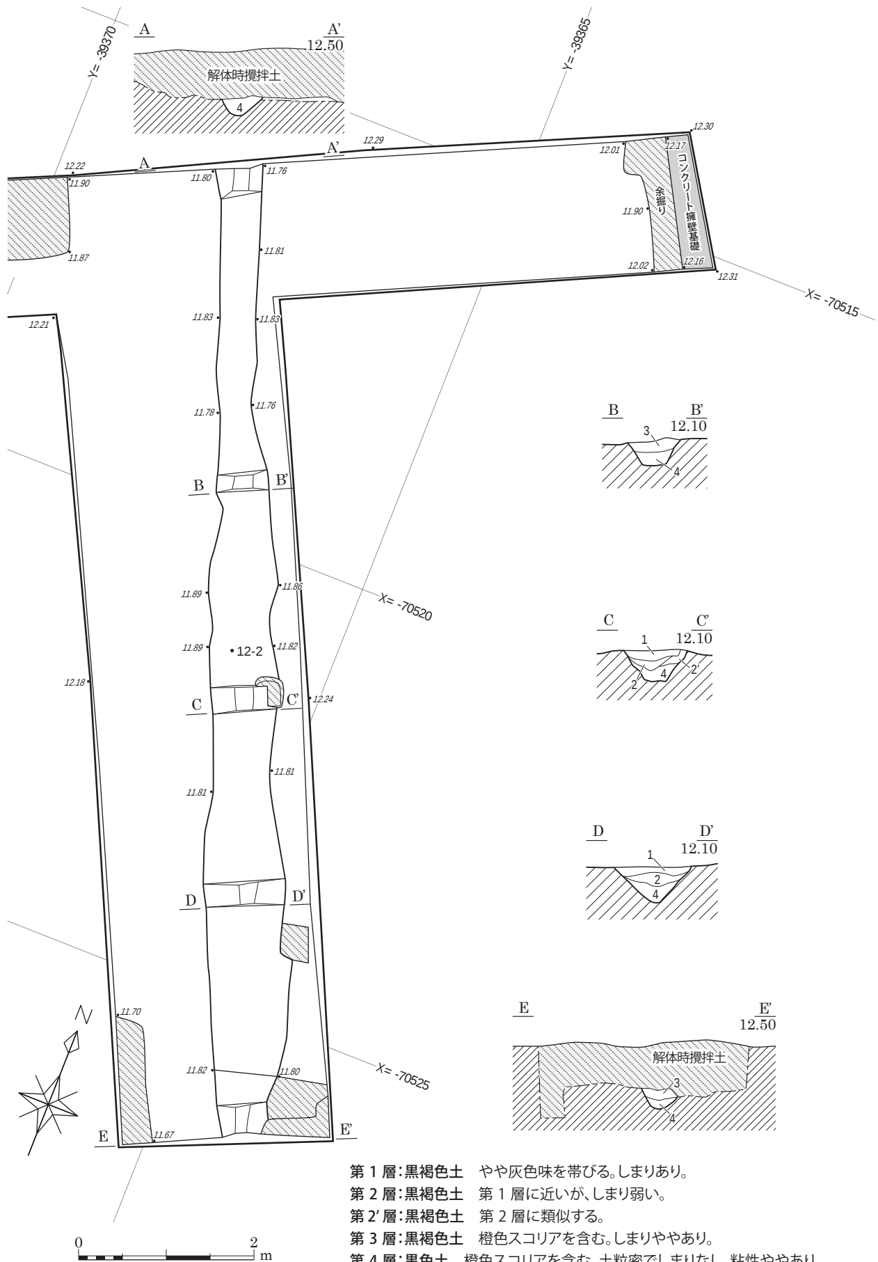
第 11 図 溝状遺構平断面図 (1/60)
