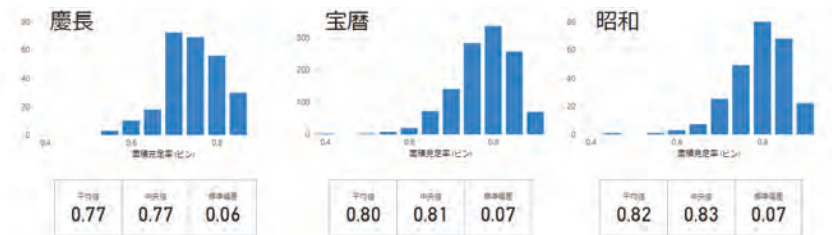
図 15 築石の矩形充填率のばらつき
