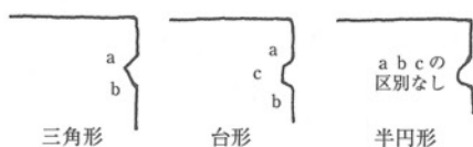
図2 切込み形状
