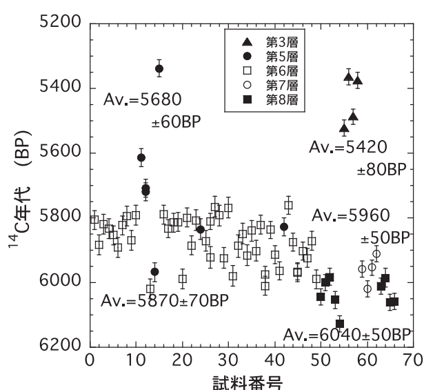
図2 田螺山遺跡出土木柱の ^{14}\text{C} 年代
