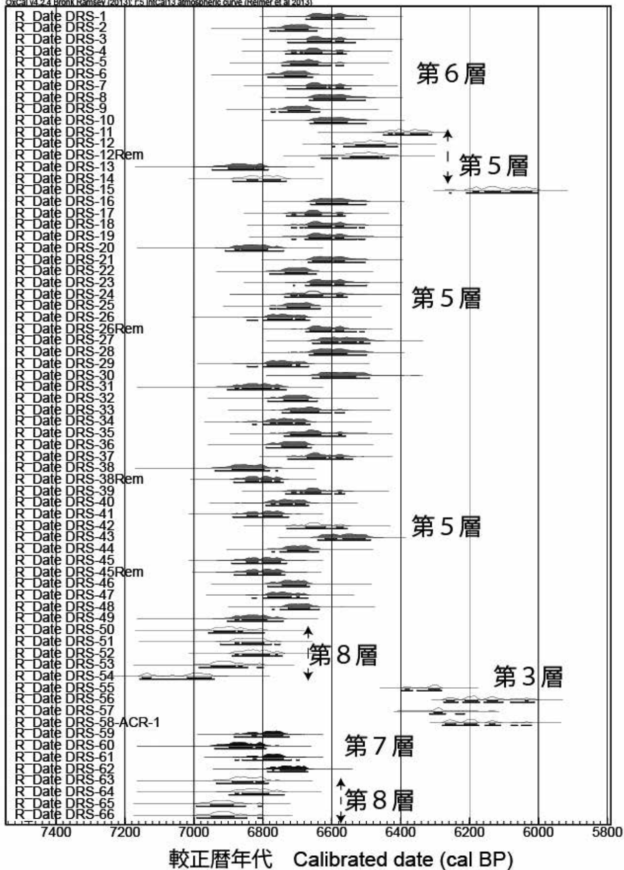
図3 田螺山遺跡出土木柱の較正暦年代 图3 田螺山遗址出土木柱的校正日历年代
