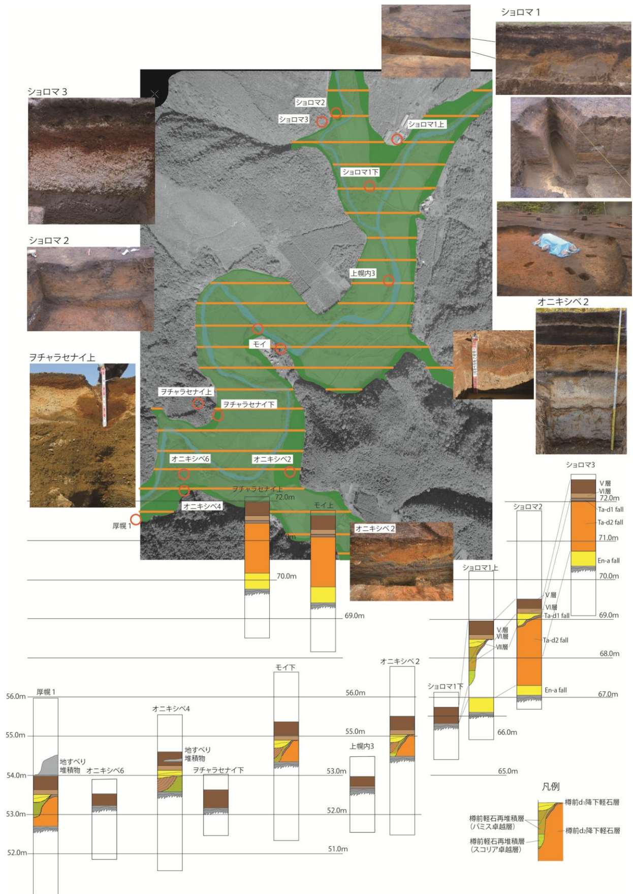
第1-3 厚真川上流域の樽前d火山灰降下後の土石流分布
