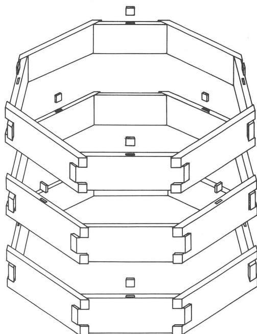
図11 井戸枠組み上げ模式図
