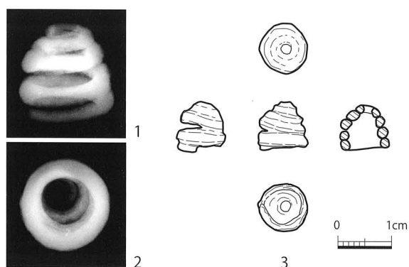
第22図 出土銅製品のX線透過写真(1、2)および実測図(3、1:1)
