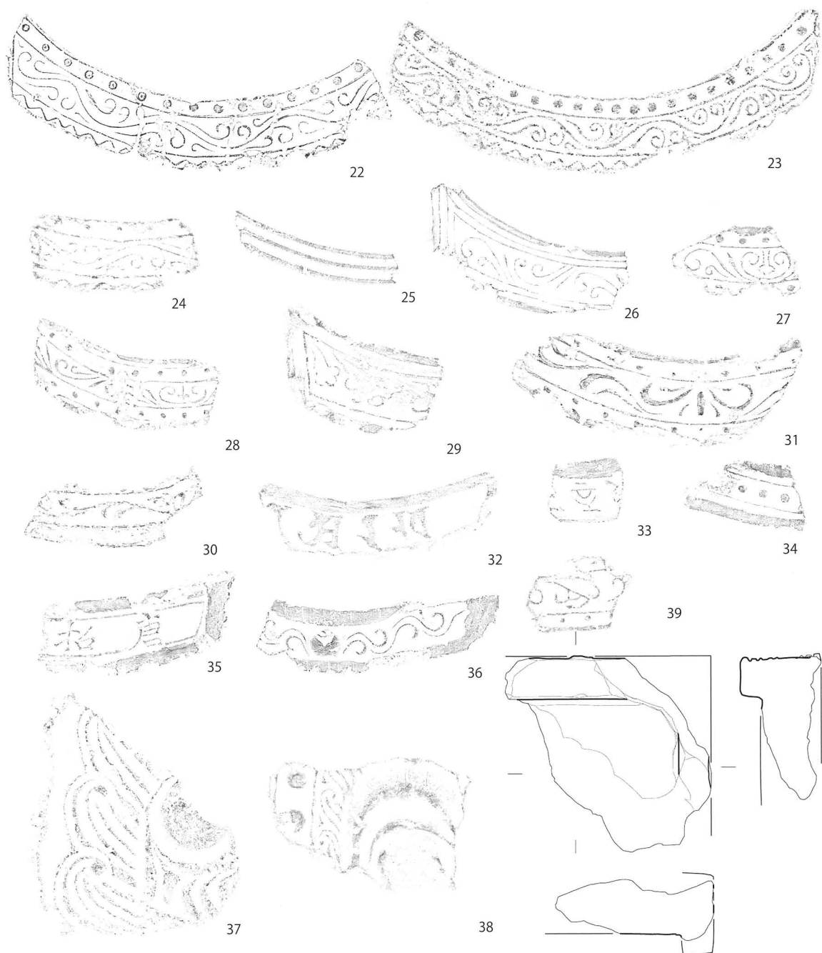
第20図 出土軒平瓦・鬼瓦・隅木蓋瓦（1：4）
