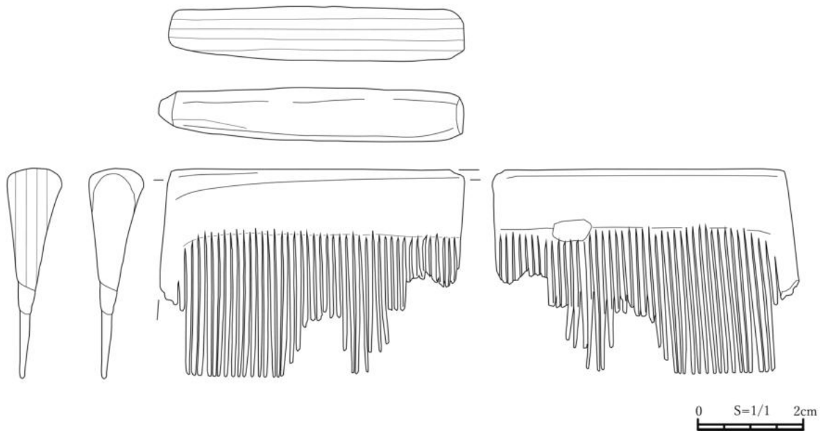
図6 櫛実測図
