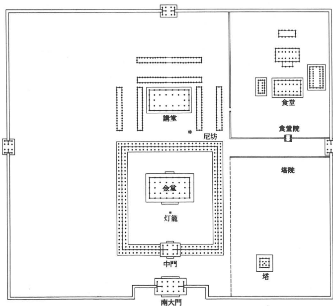
fig.25 西隆寺伽藍図 1:3000
